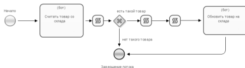
Рис. 2: Подпроцесс-композиция обновления остатка
