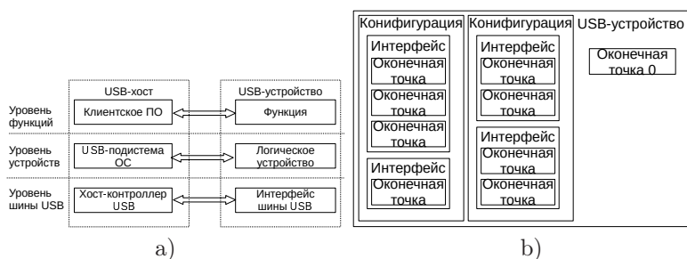
Рис. 1: Уровни организации интерфейса USB (а) и иерархическое представление USB-устройства (б)
