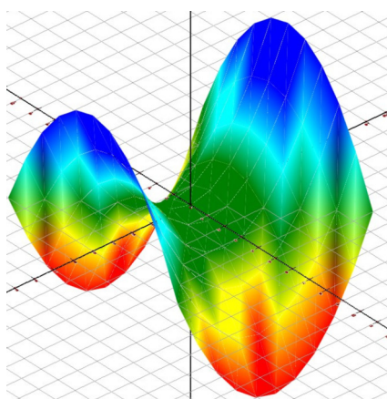
Рис. 3: Пример поверхности
