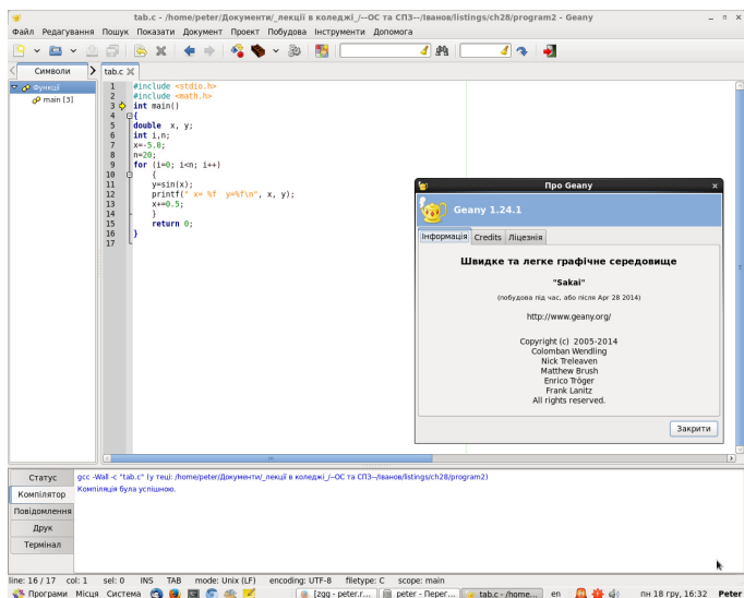
Рис. 2: Оболочка Geany
